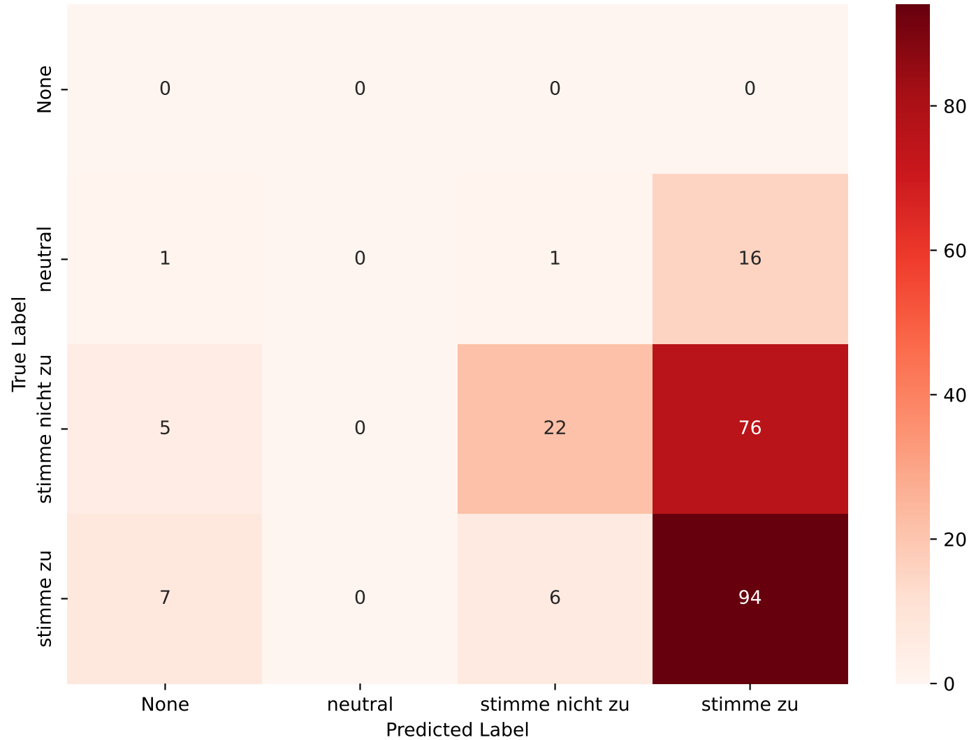
Confusion Matrix - Llama 2, temp: 0.1
